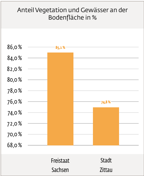
Abb. 25: Anteil Vegetation und Gewässer an der Bodenfläche in %
